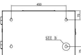
Zadní pohled
