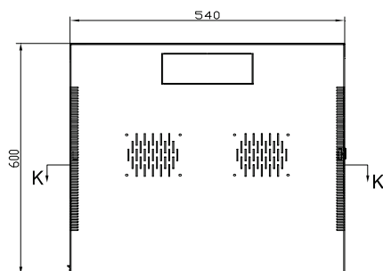
Vrchní pohled
