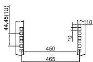
Montážní rozměry
