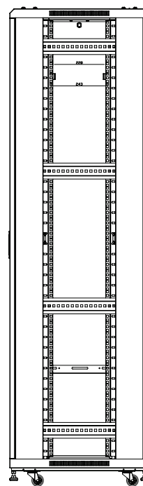
Boční pohled (bez dveří)
