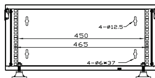
Řez K-K
