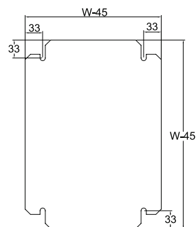
Montážní panel
