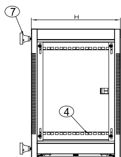
Boční pohled (bez bočního panelu)
