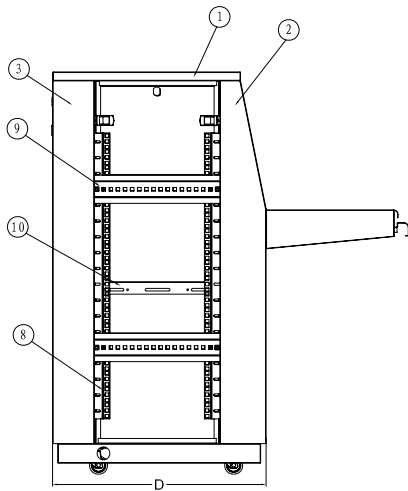
Boční pohled (bez bočního panelu)
