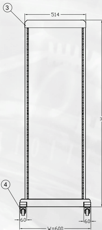
Řez A-A
