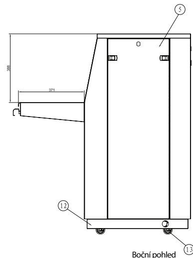
Boční pohled
